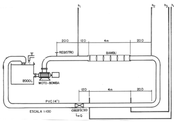
Figura 1 – Bancada para ensaio de perda de carga
