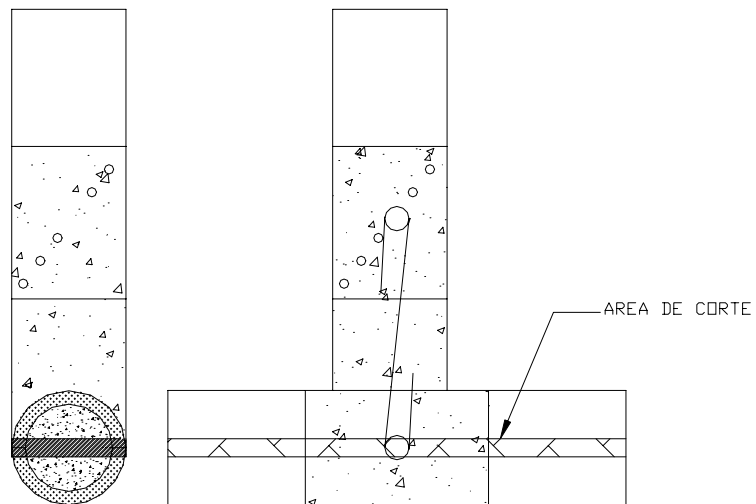
FOTO 43 FALLA UNION DG 90° TENSION
