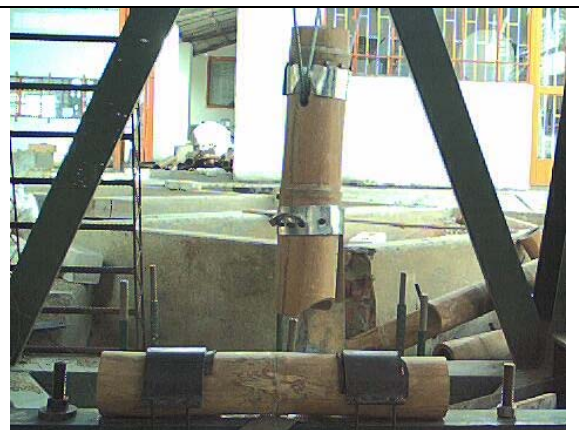
FOTO 29 FALLA UNION SC 90° TENSION
